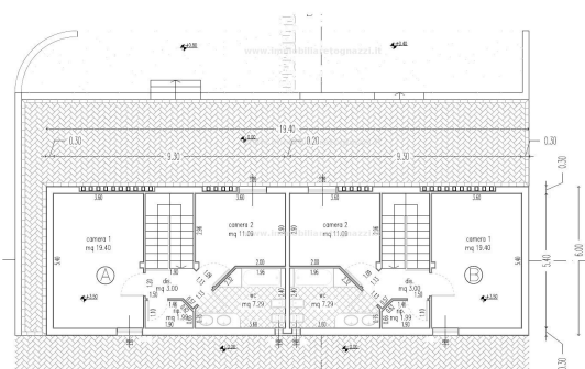
IPOTESI DI PROGETTO PER LA REALIZZAZIONE DI N.2 UNITA' TERRATETTO AD USO ABITAZIONE PIANO PRIMO ED ULTIMO
