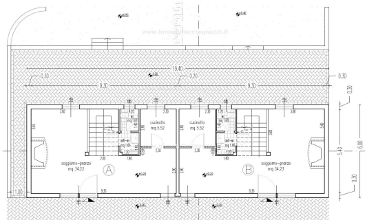
IPOTESI DI PROGETTO PER LA REALIZZAZIONE DI N.2 UNITA' TERRATETTO AD USO ABITAZIONE PIANO TERRA
