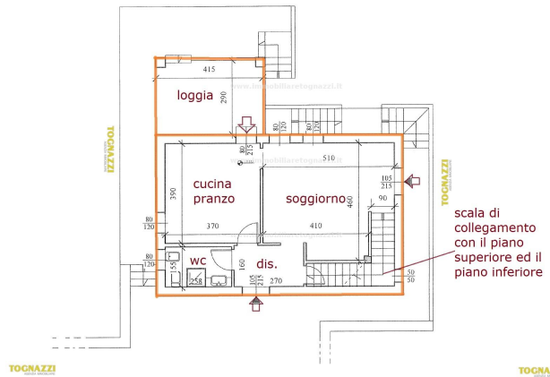
PIANO TERRA ipotesi di progetto
