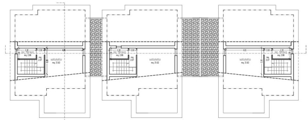
PIANTA PIANO SOTTOTETTO rapp. 1:100
