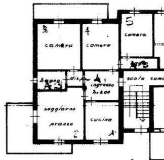
PIANO RIALZATO
