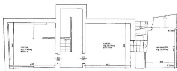
PIANTA PIANO INTERRATO
