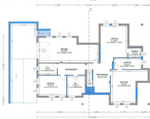
pianta piano seminterrato
