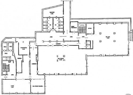
PIANTA PIANO SEMINTERRATO
