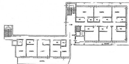
PIANTA QUARTO PIANO
