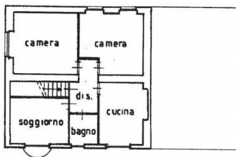
PIANO PRIMO h=295 cm
