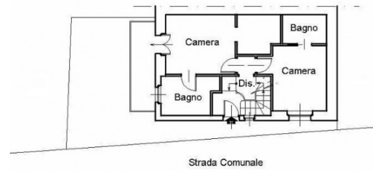
PIANTA PIANO TERRENO H = 255 cm
