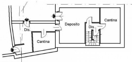
PIANTA PIANO SOTTERRANEO H = 255 cm
