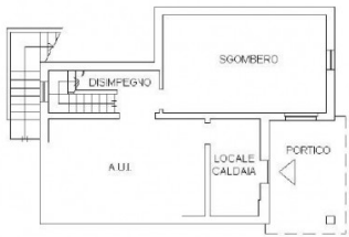
PIANO PRIMO INTERRATO
