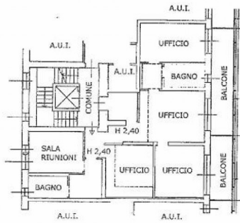
PIANO SECONDO H 2,70
