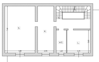
PIANTA PRIMO PIANO
