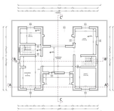
PIANTA PIANO TERRENO Scala 1:100
