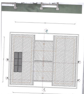
PIANTA COPERTURA TETTO CAPITANTE 3 KW Scala 1:100
