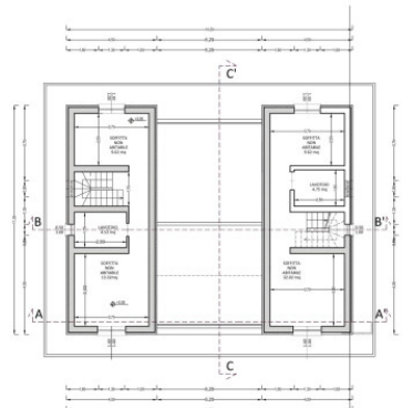
PIANTA PIANO SOTTOTETTO Scala 1:100
