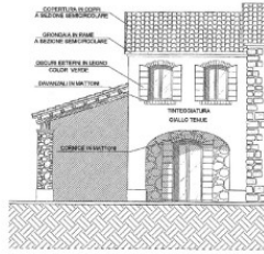
PARTICOLARE COSTRUTTIVO
