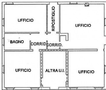
PIANTA PIANO TERRA H=284
