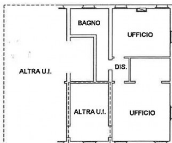
PIANTA PIANO PRIMO H=300
